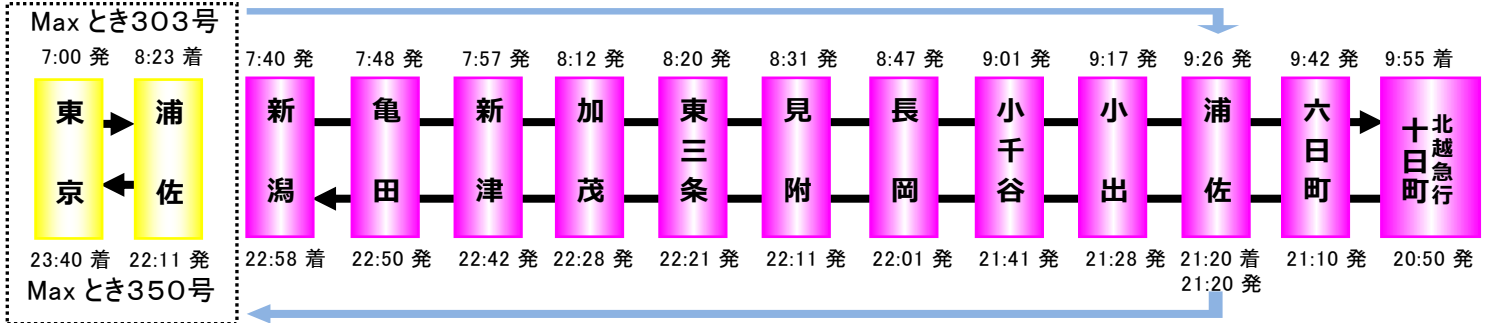
E653系車両
